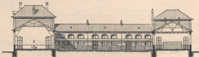
Querschnitt.
