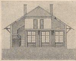
Querschnitt.
