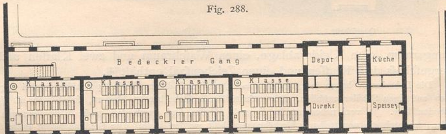
Obergeschoss.
