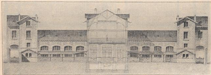
Querschnitt durch den Spiel- und Zeichenfaal und Rückansicht der Kleinkinderschule.
