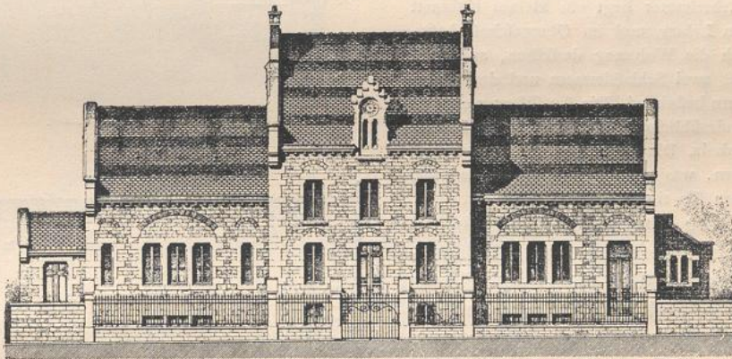
Hauptansicht. — \frac{1}{350} w. Gr.
