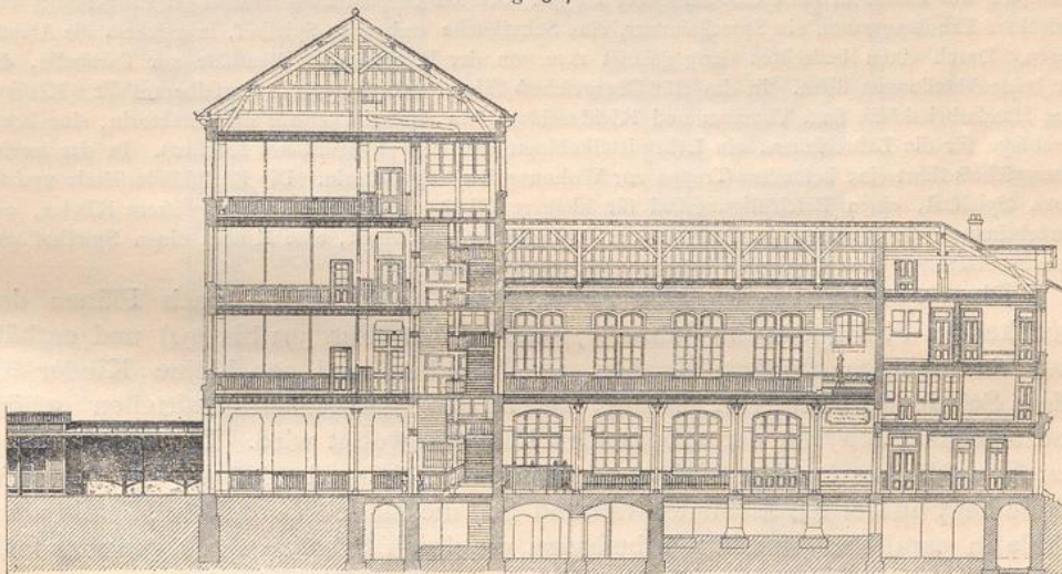
Querfchnitt durch die Mitte.
