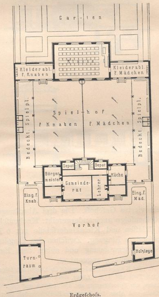
Erdgeschoß. Einklassige gemischte Volksschule und Gemeindeamt zu Gouillons (Eure et Loir) . — \frac{1}{500} w. Gr.
