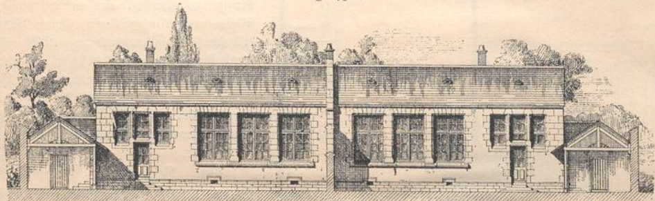
Anficht des Klassenhauses.
