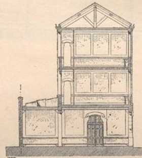
| Querschnitt durch die Knabenschule.
