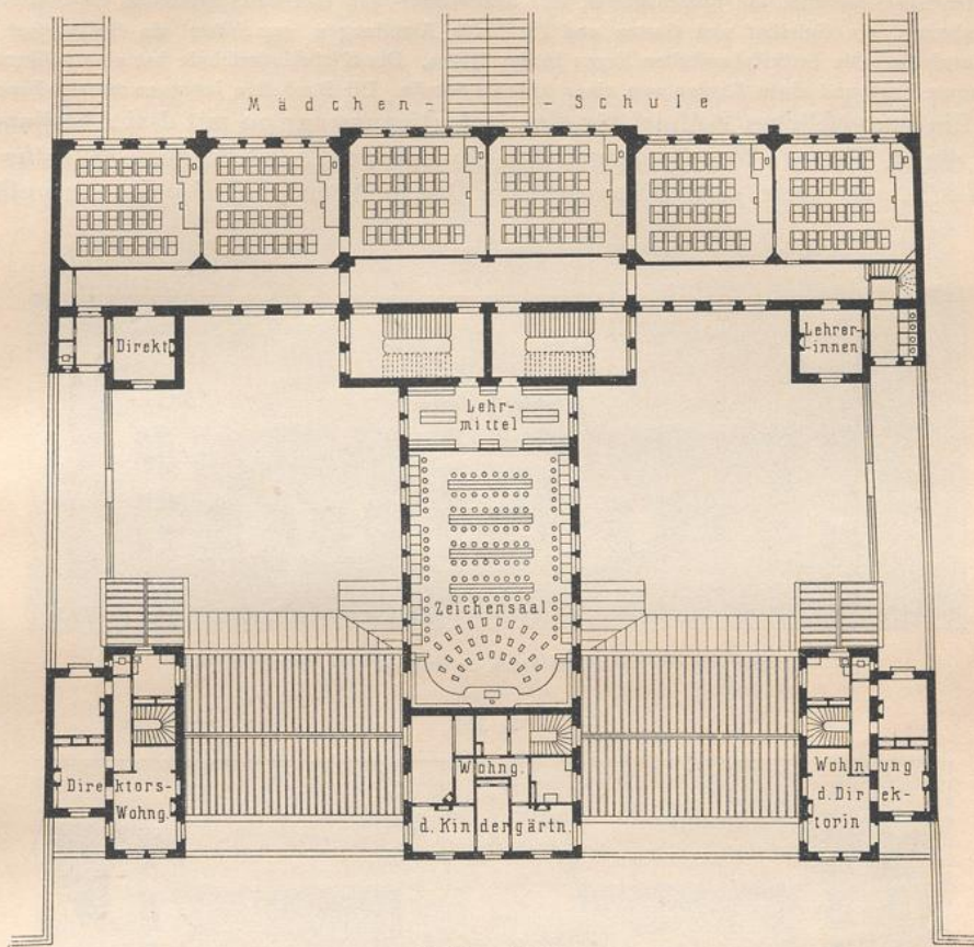
I. Obergechois.
