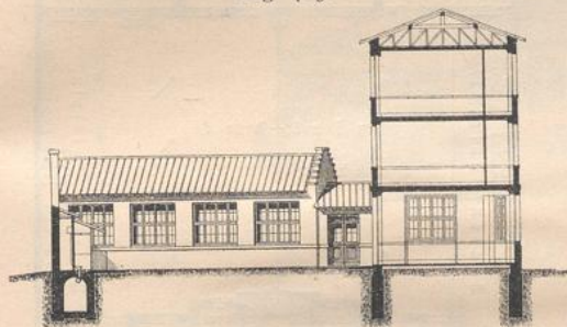
Querschnitt durch die Kleinkinderschule. Schulhausgruppe zu Paris, Rue Brodu.
