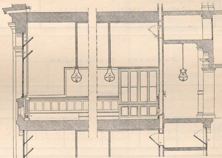
Einzelschnitt durch Lehrzimmer und Gang zu Fig. 341 bis 345.
