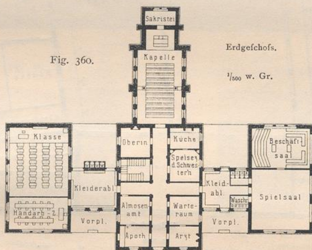
Mädchen- und Kleinkinderschule zu Fontaines (Saone-et-Loire) .
