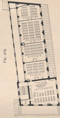
I. Obergeschoss der Knabenschule.
