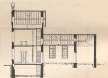
Querschnitt
