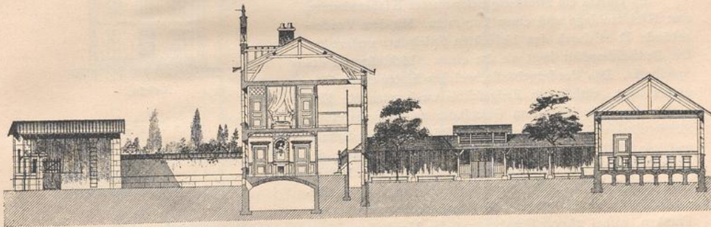
Querschnitt durch die Mitte. — \frac{1}{275} w. Gr.
