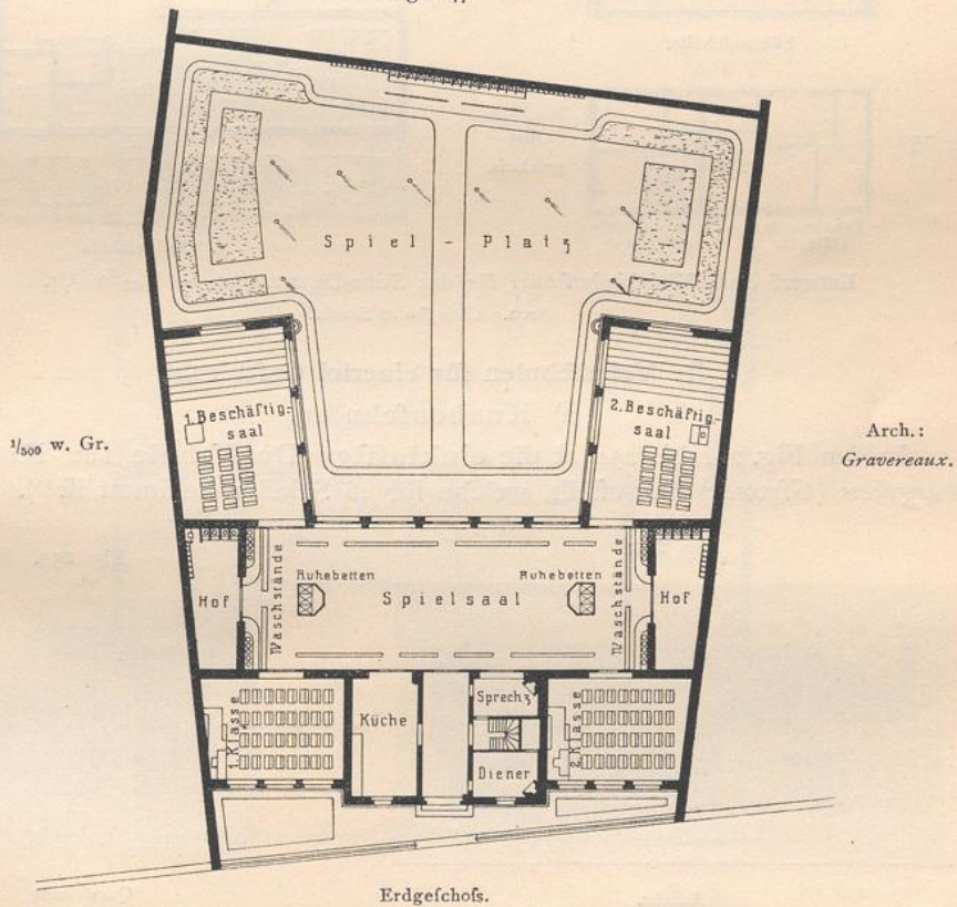
Kleinkinderschule zu Charenton.
