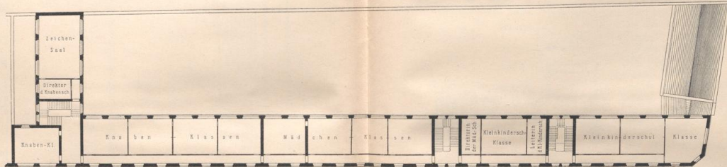
I. Obergeschoss.
