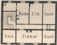
Obergeschoss.
