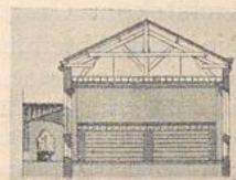
Schnitt durch den Beschäftigungssaal.
