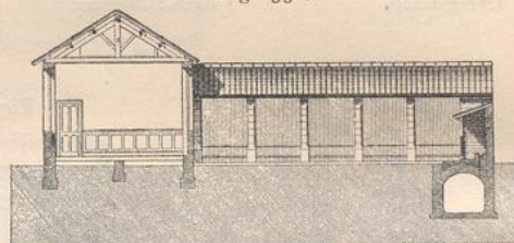
Querschnitt. — 1/375 w. Gr.
