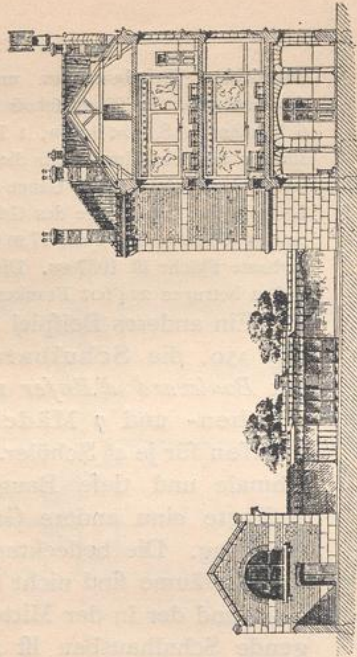
Querfchnitt.
