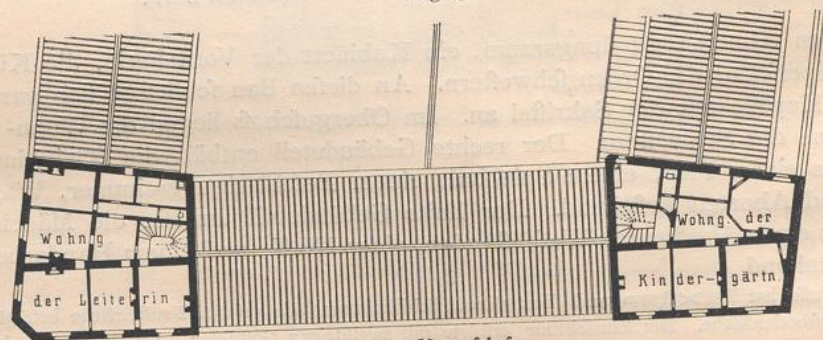
Mädchen- und Kleinkinderfchule
