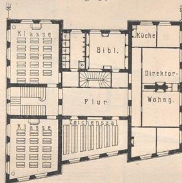
Obergeschoss.
