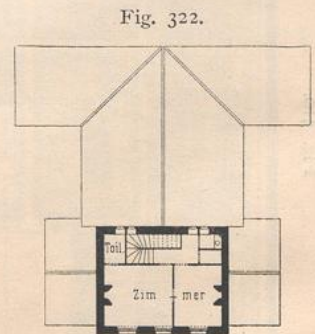
Obergeschofs.
