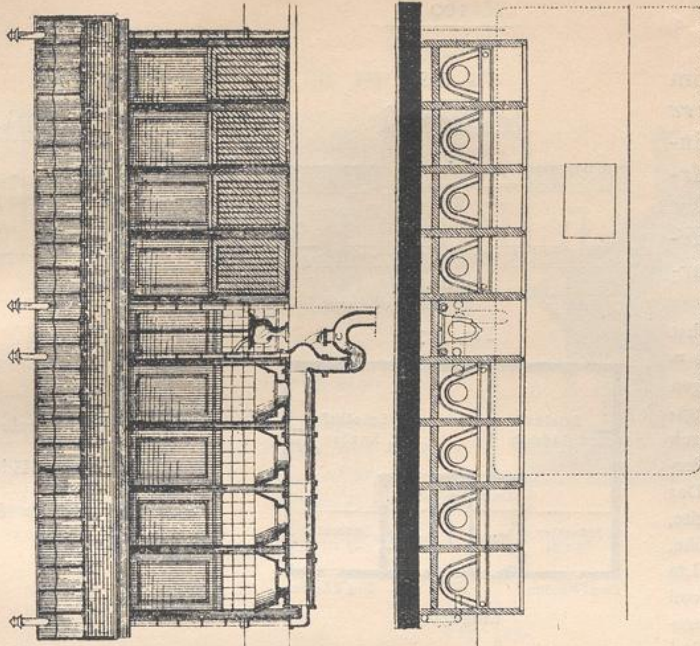
Ansicht u. Grundriss.
