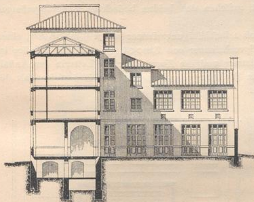
Querschnitt durch das Klaffengebäude für Knaben.
