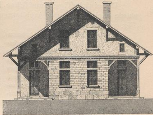
Ansicht. — \frac{1}{250} w. Gr.
