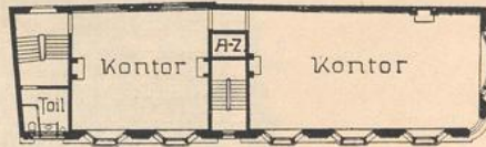
I. Obergeschoss.
