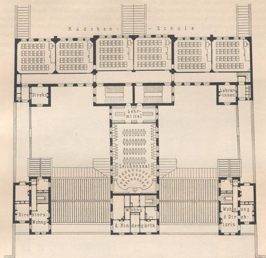
I. Obergechois.
