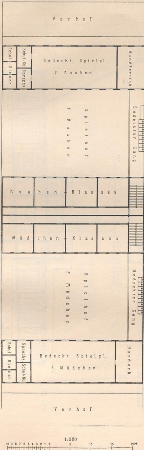
Grundriss der 14klassigen Schulbaracke zu Paris, Boulevard d'Enfer. Arch.: Bonvard.
