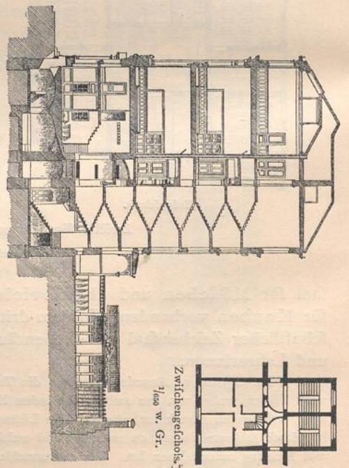
Fig. 342.
