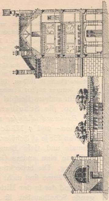
Querfchnitt.
