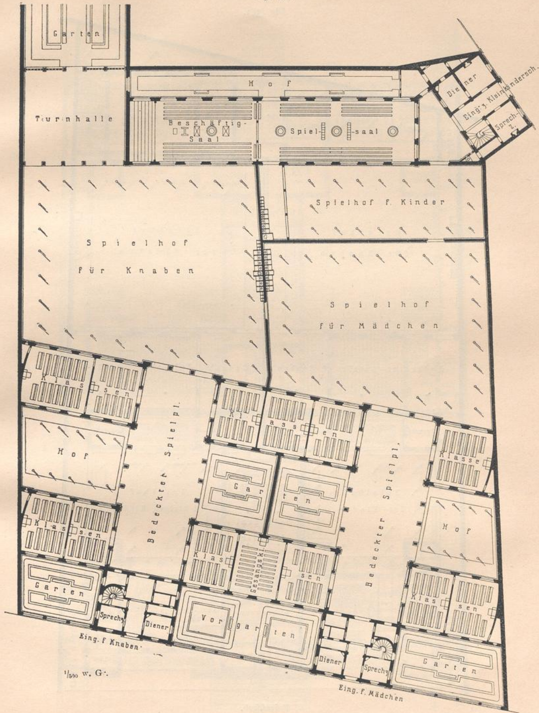
Fig. 380.
