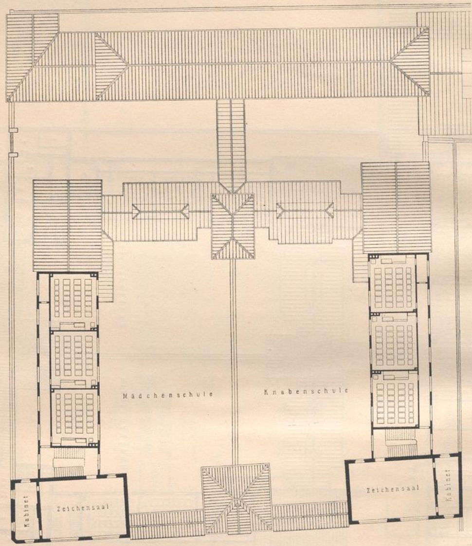
Fig. 409.
