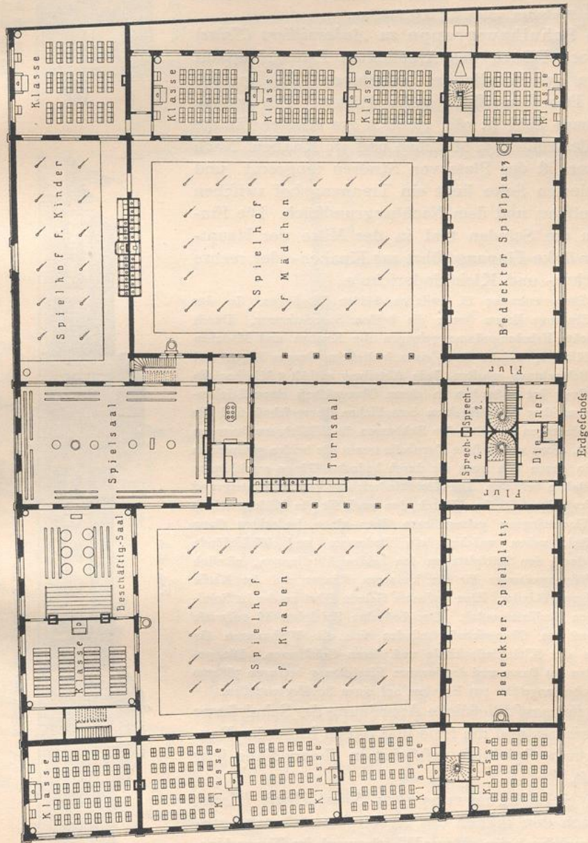
Schulhausgruppe zu Aubervilliers (Seine).
