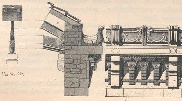
Querschnitt durch den bedeckten Spielplatz,
