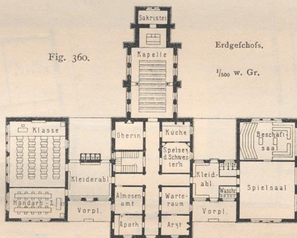
Mädchen- und Kleinkinderschule zu Fontaines (Saone-et-Loire) .
