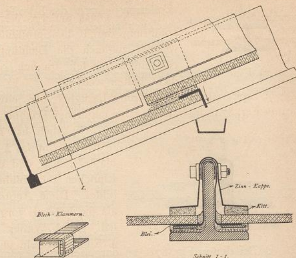
Glasdeckung von Göller 153 . 1/2 n. Gr.
