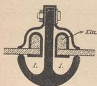
Sproffen von Drummond 153) . 1/2 n. Gr.
