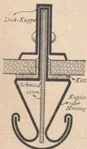
Sprosse System Hayes 153 , 1/2 n. Gr.
