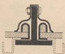
Sproffen von Drummond 153) . 1/2 n. Gr.
