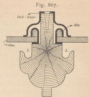
Sprosse von Drummond 153 ), 1/2 n. Gr.
