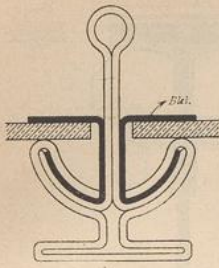
Sprossen von Pennycook 153 , Nat. Gr.
