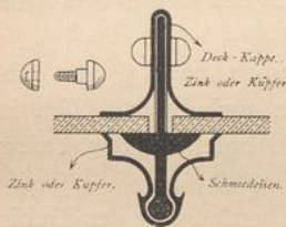
Sprosse von Shelley, (System Unique 153 ), 1/2 n. Gr.
