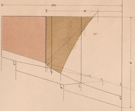
Vertical-Schnitt.
