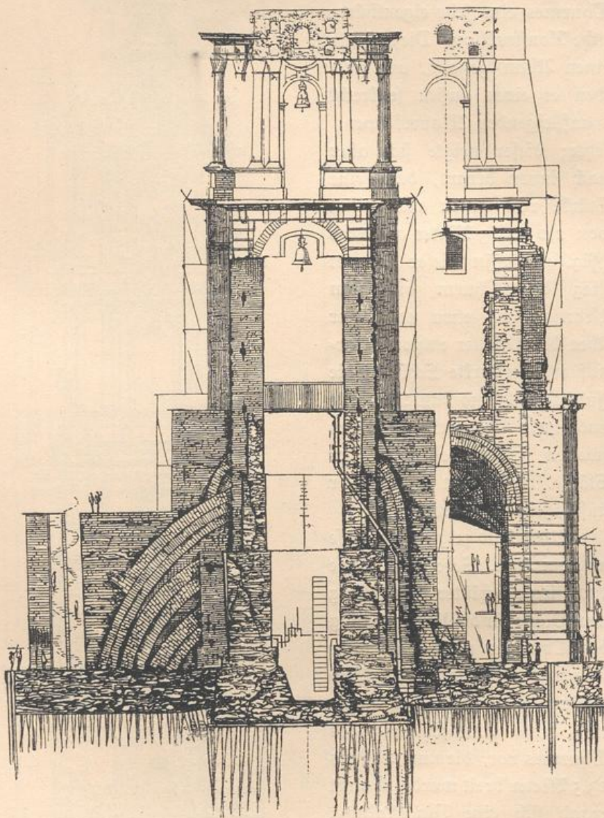
fig. 48. Broebes' Skizze zum Bau des Münzthurmes.
