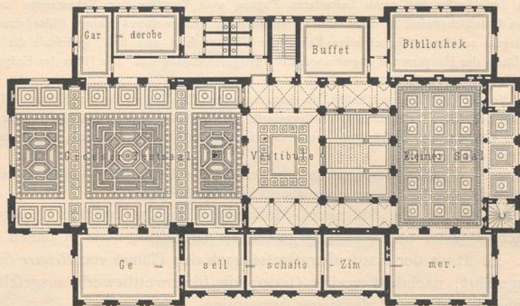
Obergeschoss.
