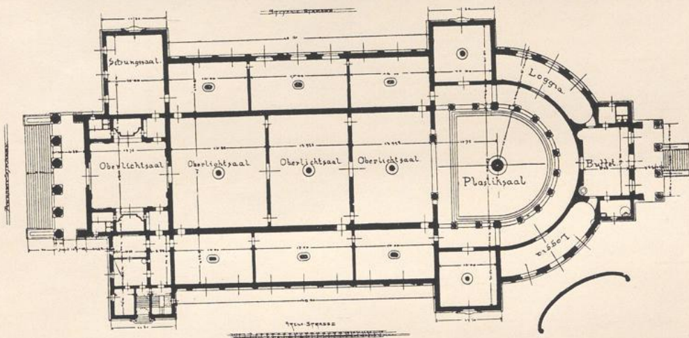
Grundriss.
