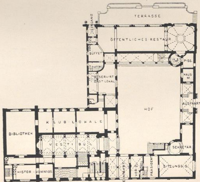
Grundriß des Erdgeschosses. 1/1000 w. G.
