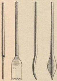
Werkzeuge für Ausführung des Sgraffito 139) .
