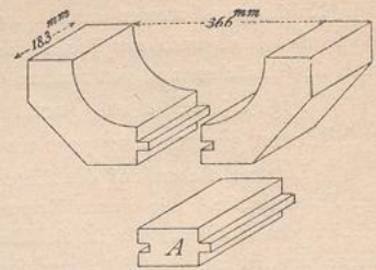
Krippen-Einfätze.
