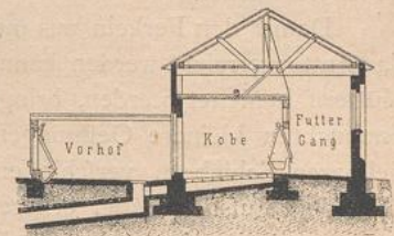
Fig. 121. Querschnitt des Schweineftalles in Fig. 120. 1/200 n. Gr.
