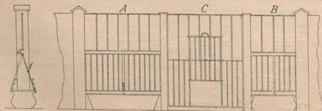
Kobwand aus beweglichem Gitterwerk. — 1/50 n. Gr.
