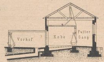
Fig. 121. Querschnitt des Schweinefstalles in Fig. 120. 1/200 n. Gr.
