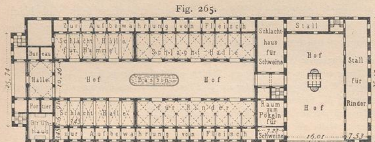
Schlachthof zu St. Lorenzo bei Genua 108 ). — 1/1000 n. Gr.
