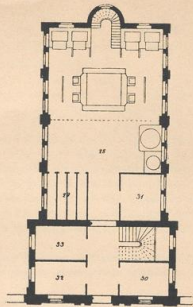
Wasch- (und Bade-) Anstalt für Arme. 1:250
