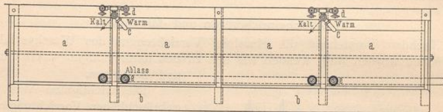
Handwaschbottiche für öffentliche Waschlhäuser von Gebr. Foensgen zu Düsseldorf. Ansicht von oben. — \frac{1}{25} w. Gr.
