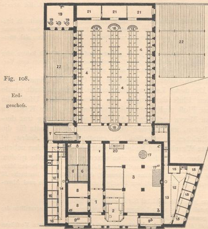
Wasch- (und Bade-) Anstalt in der Kapuzinerstrasse zu Metz 34) .
