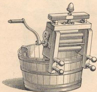
Wringmaschine für Handbetrieb 19) .
