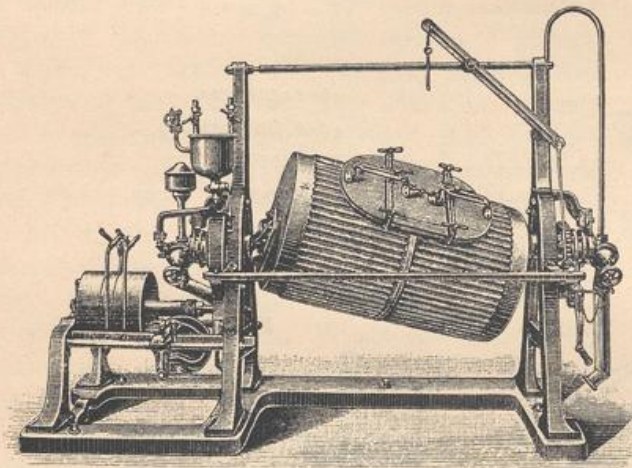
Ansicht.
