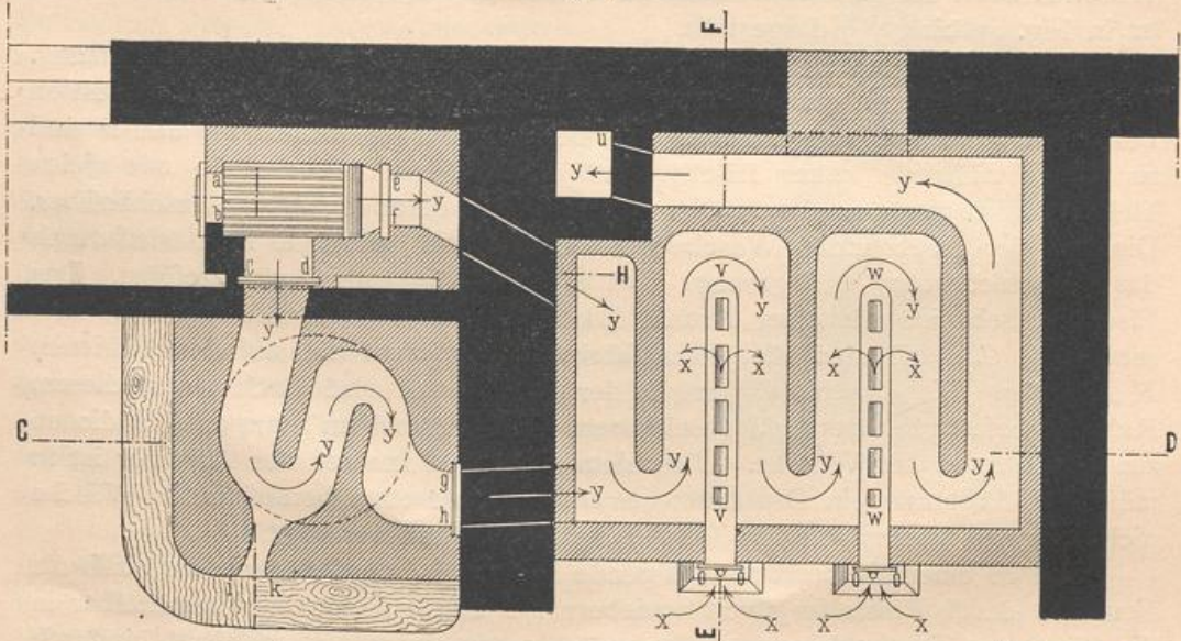
Wagrechtter Schnitt nach AB in Fig. 45 (nahe am Fußboden).
