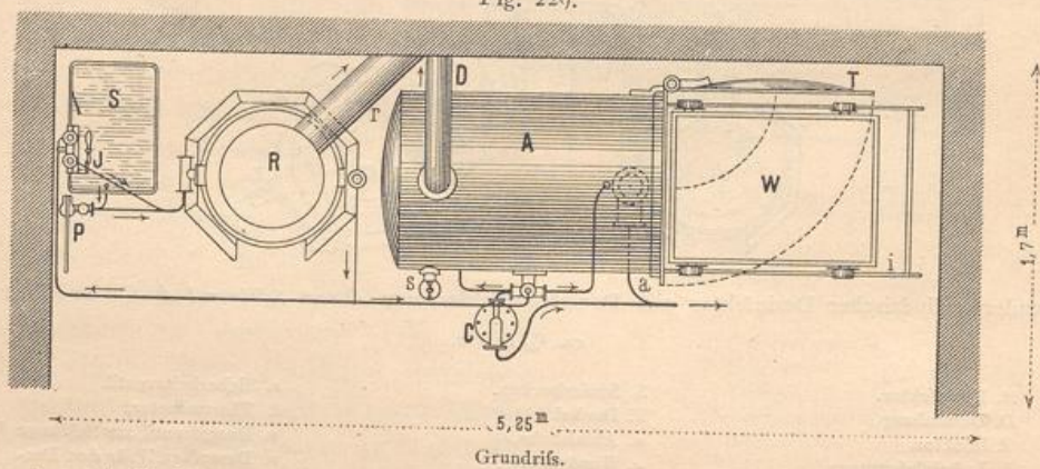
Grundriß.
