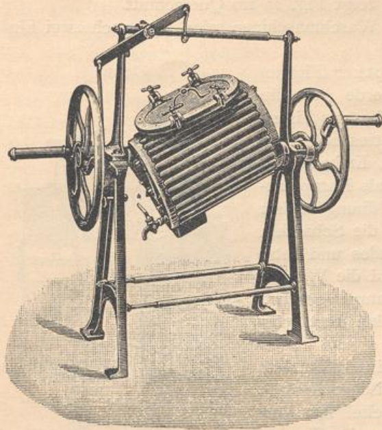
Einfache Trommel-Waschmaschine für Handbetrieb von Oscar Schimmel & Co. zu Chemnitz. \frac{1}{25} w. Gr.
