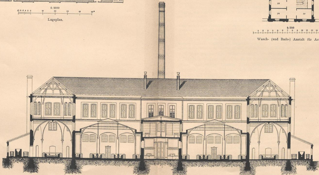
Öffentliche Wasch- (und Bade-) Anstalt zu Caën. Schnitt. 1:250
