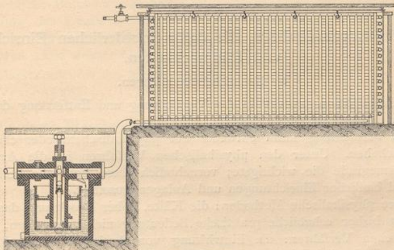
Längenschnitt.
