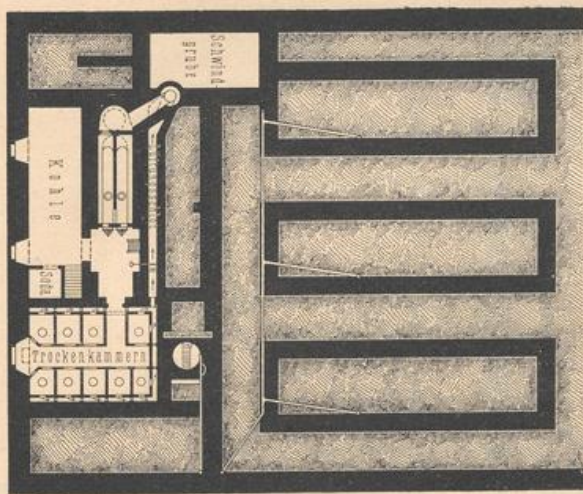
Kellergeschofs.
