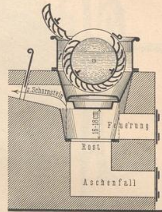
Dampfwaschkessel „Neptun“ (Patent Hoese ) von Kurd Hahn zu Berlin. 1/25 w. Gr.
