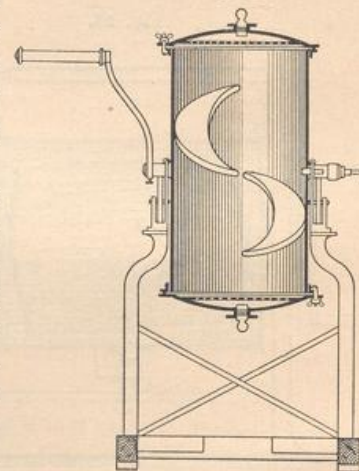
Wasch- und Spülmaschine „Blanka“ (Patent Hoese ) von Kurd Hahn zu Berlin. 1/50 w. Gr.
