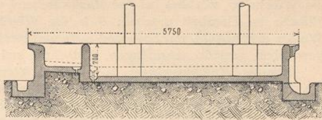
Längenschnitt.
