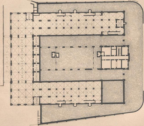
Grundriss des Kellergeschosses.
