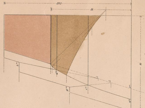
Vertical-Schnitt.
