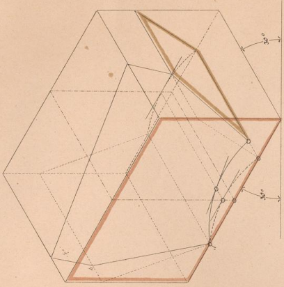
Schlusstein.
