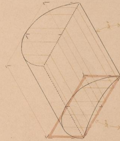
Isometrische Projection des Trompillons.
