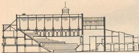
Längenschnitt.
