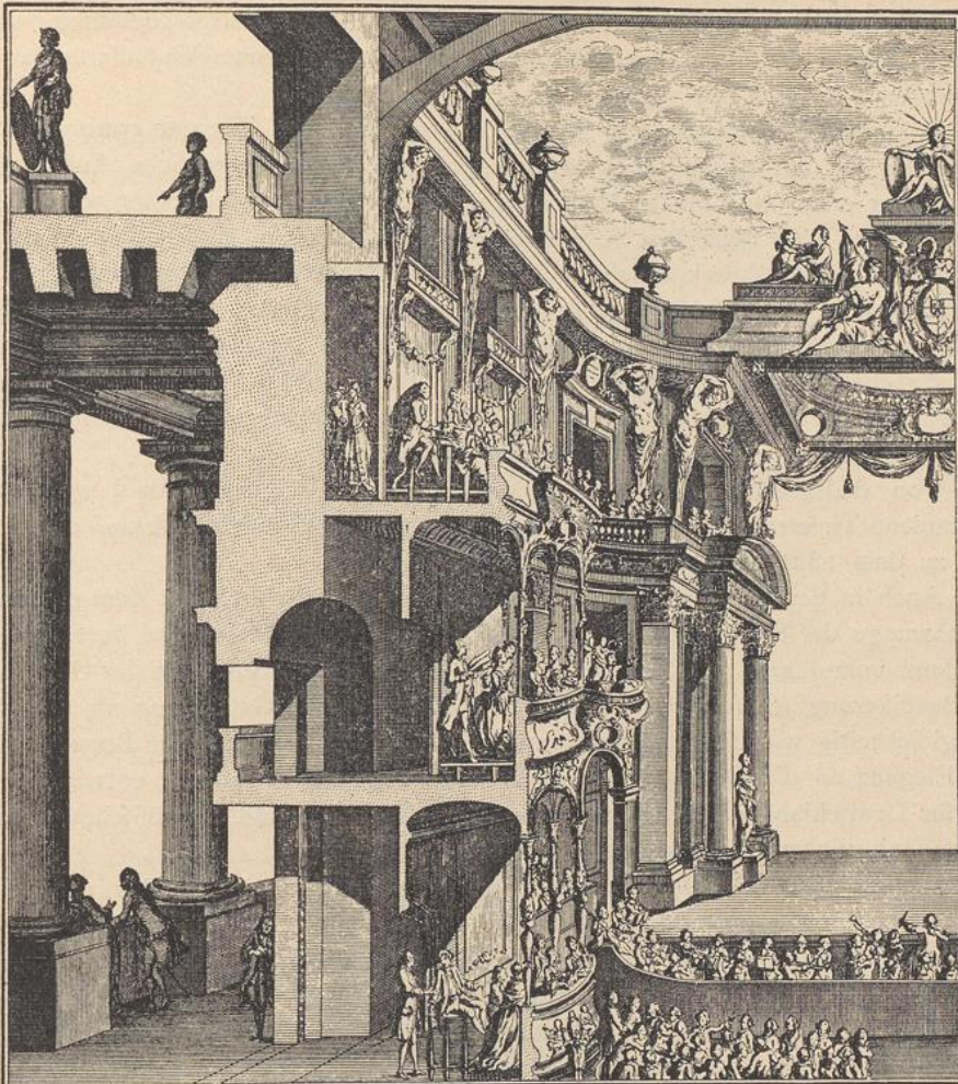
Coupe du nouvel Opéra de Stuttgart esquisse pour en voir l'effet sans aucunes règles de Perspective.
