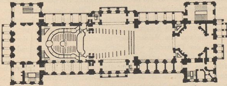
Plan où Projet de la restauration de l'Opéra de Stuttgart.
