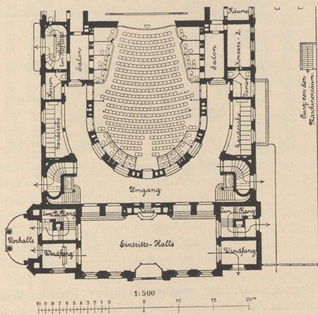
Parterregrundriß 75).
