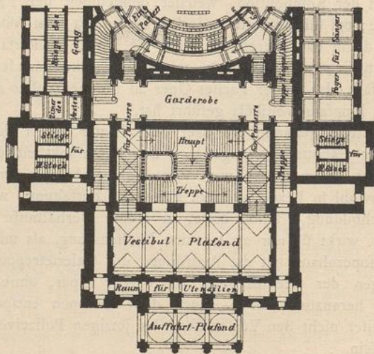
Königl. Opernhaus zu Budapest 50).
