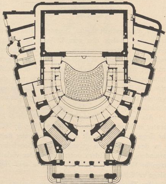
Theater zu Karlsbad 80) . Arch.: Fellner & Helmer. \frac{1}{500} w. Gr.
