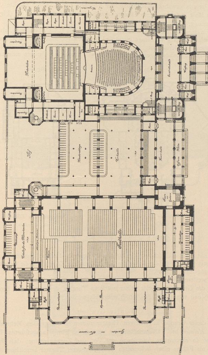
Stadttheater und Festsalle zu Nürnberg 75) .
