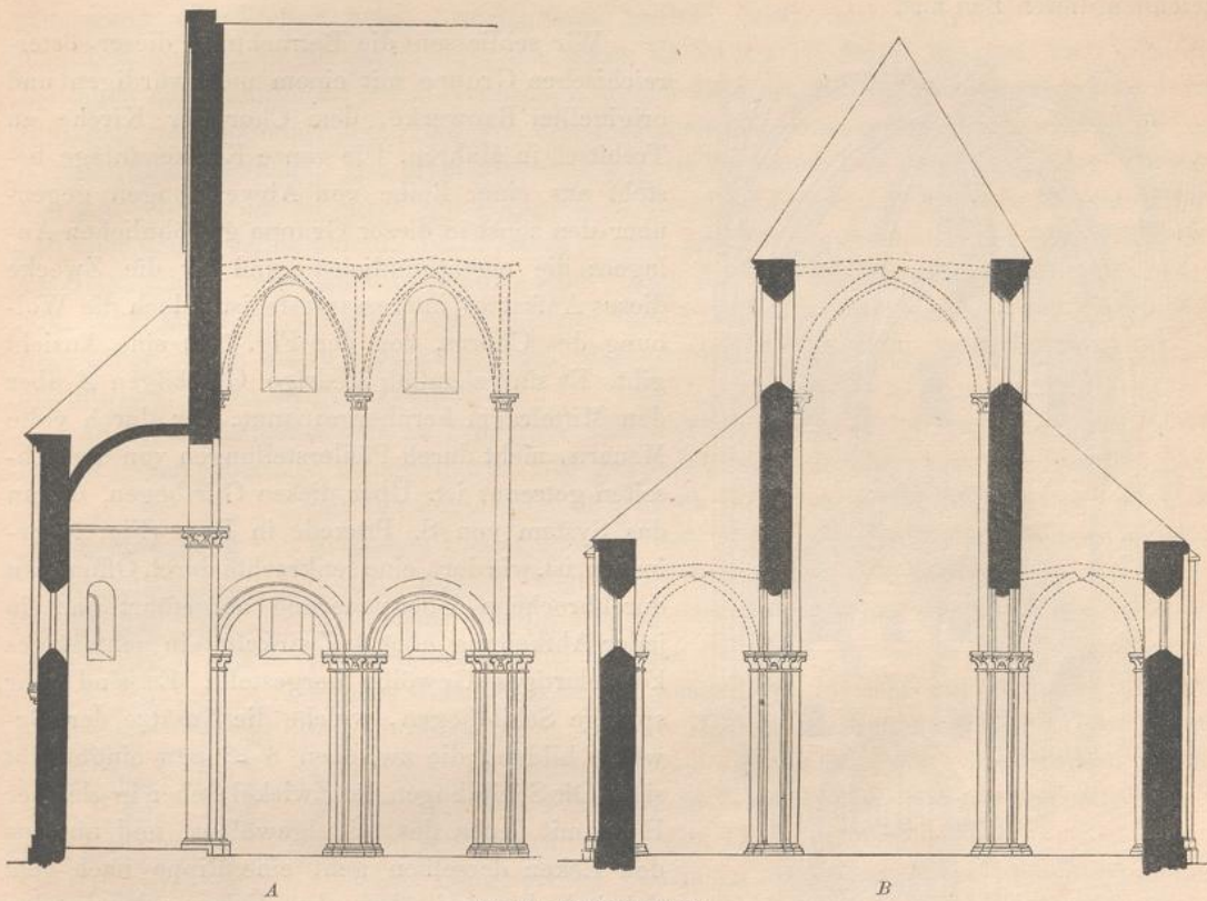
Fig. 70. Kirche zu Lébeny.
