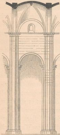
Fig. 68. Joch aus dem Dome zu Trient.
