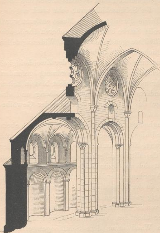
Fig. 48. System der Abteikirche zu Heisterbach.
