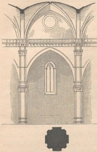
Fig. 67. Joch aus dem Dome zu Florenz.
