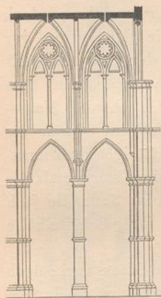
Fig. 72. Aus der Marienkirche zu Trier.
