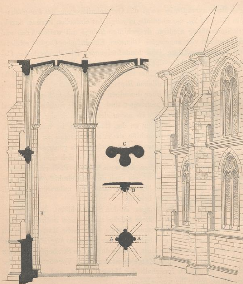
Fig. 77. Querdurchschnitt und Aussensystem der Elisabethkirche zu Marburg.
