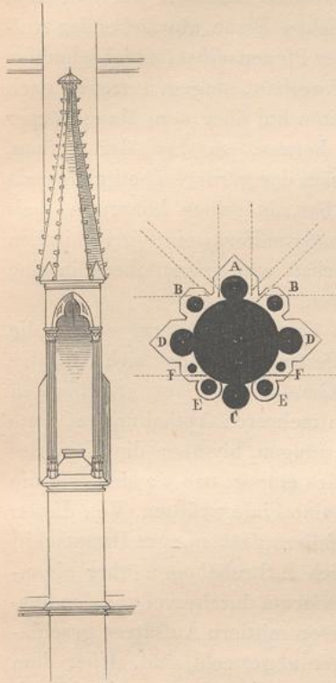
Fig. 74. Vom Dom zu Halberstadt.
