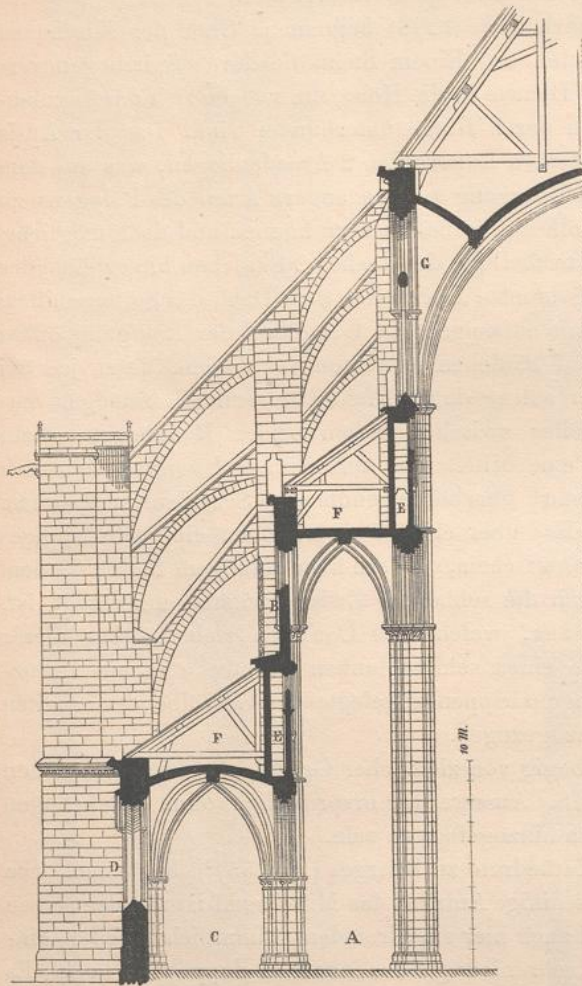
Fig. 55. Querschnitt der Kathedrale zu Bourges.
