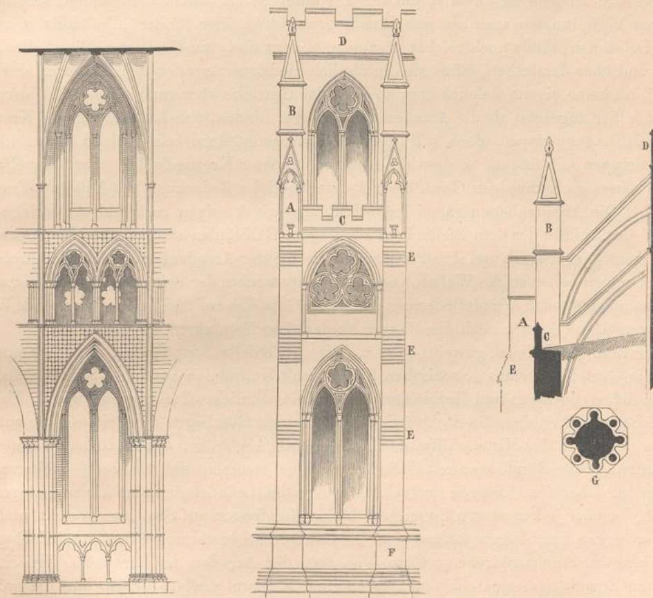
Fig. 65. Joch aus der Westminster-Abtei zu London.
