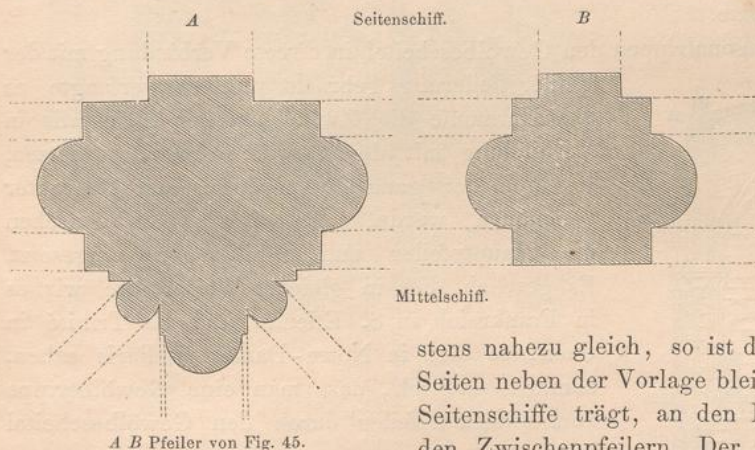
A B Pfeiler von Fig. 45.
