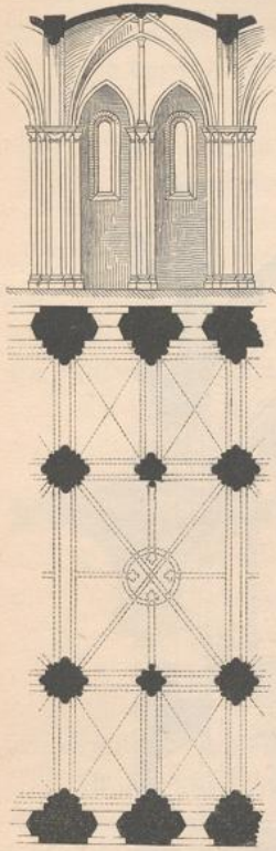
Fig. 50. Joeh aus der Kirche zu Billerbeck.
