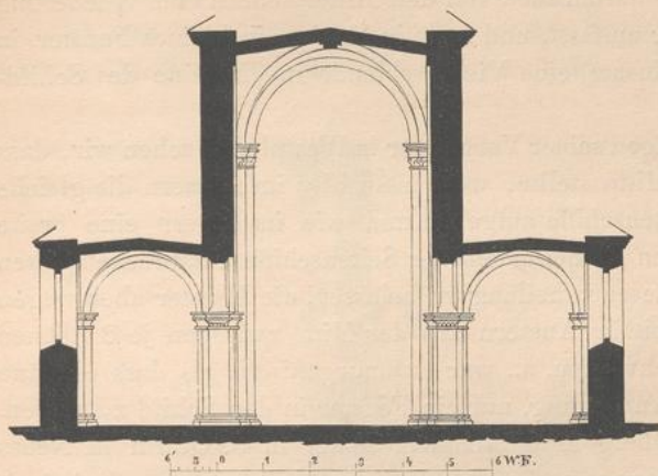
Fig. 45. Franciscanerkirche zu Salzburg. Querdurchschnitt d. Langhauses.
