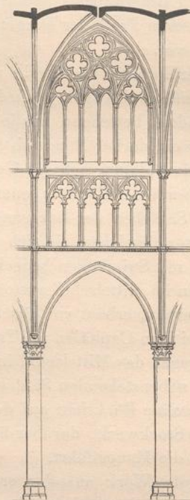
Fig. 61. Joch aus d. Langhause von S. Martin zu Ypern.
