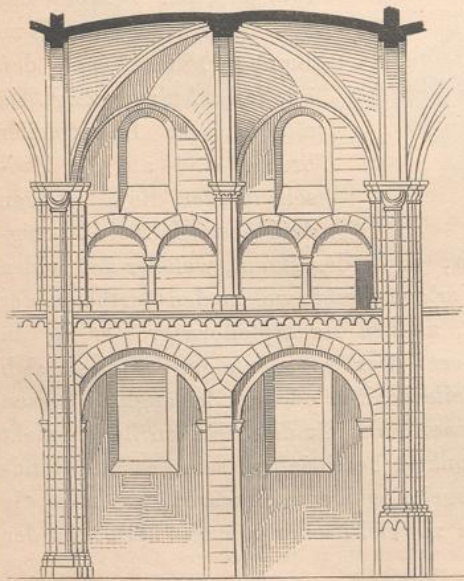
Fig. 46. Joch aus der Apostelkirche zu Cöln.
