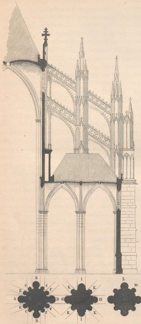
Fig. 75. Querdurchschnitt vom Chore des Domes zu Cöln (Südseite).
