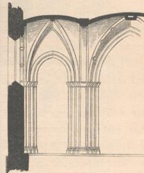
Fig. 51. Querdurchschnitt der Kirche zu Methler.
