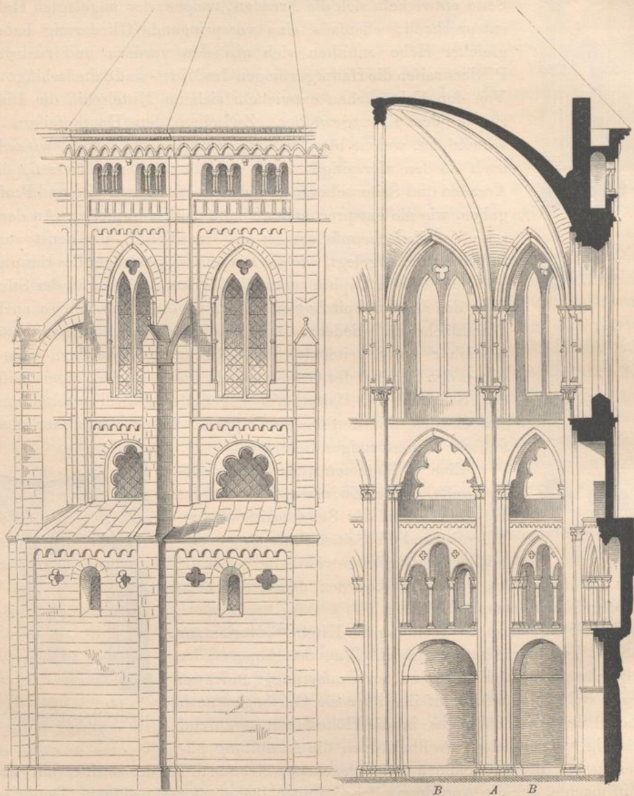
Fig. 52. Von S. Gereon zu Cöln.
