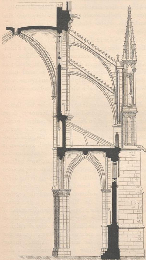
Fig. 57. Querschnitt der Kathedrale zu Rheims.
