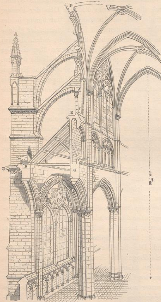
Fig. 58. Langhaus der Kathedrale zu Amiens.
