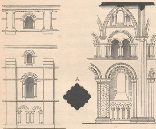
Fig. 62. Von der Kathedrale zu Durham.
