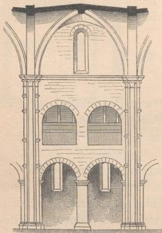
Fig. 40. Joch aus der Marienkirche zu Arnstadt.
