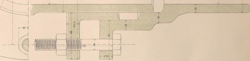
Fig. 3. Sinnatz- Muffe.
