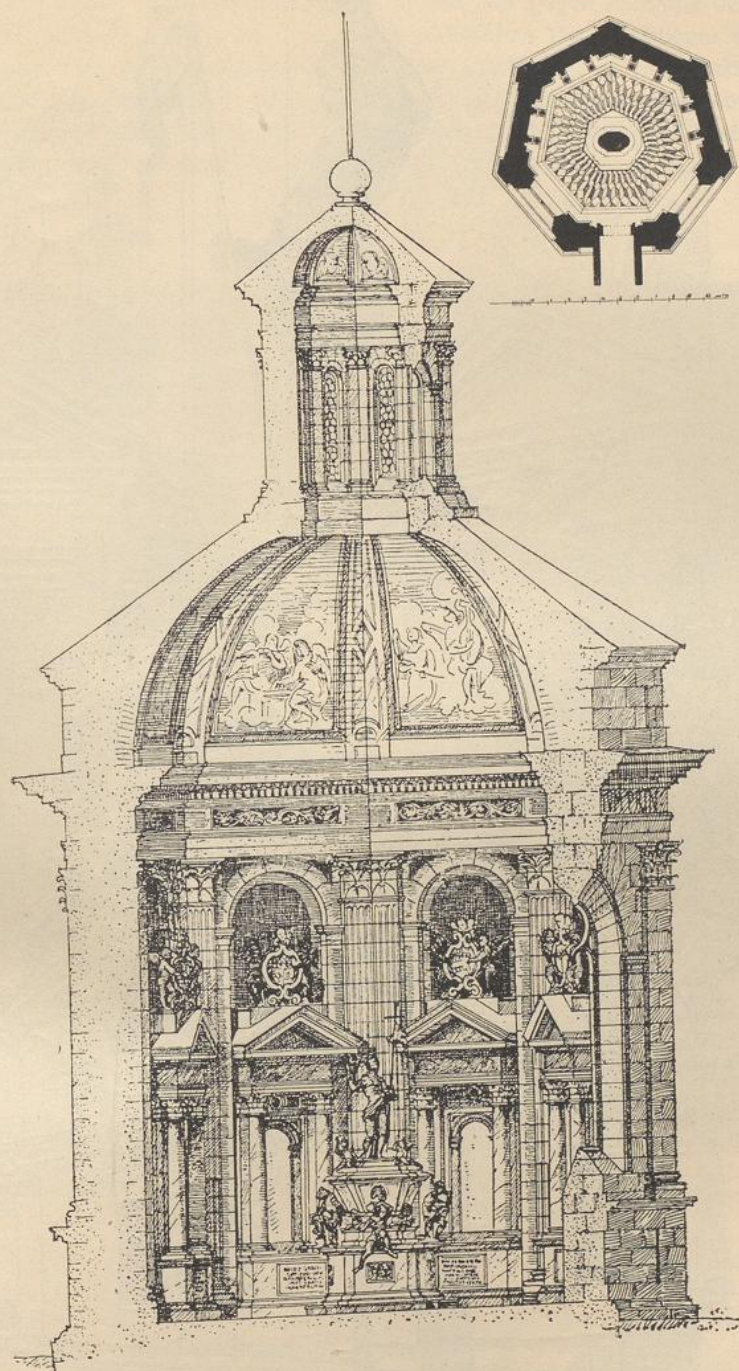
Mausoleum des Fürsten Ernst von Schaumburg zu Stadthagen 270 ).
