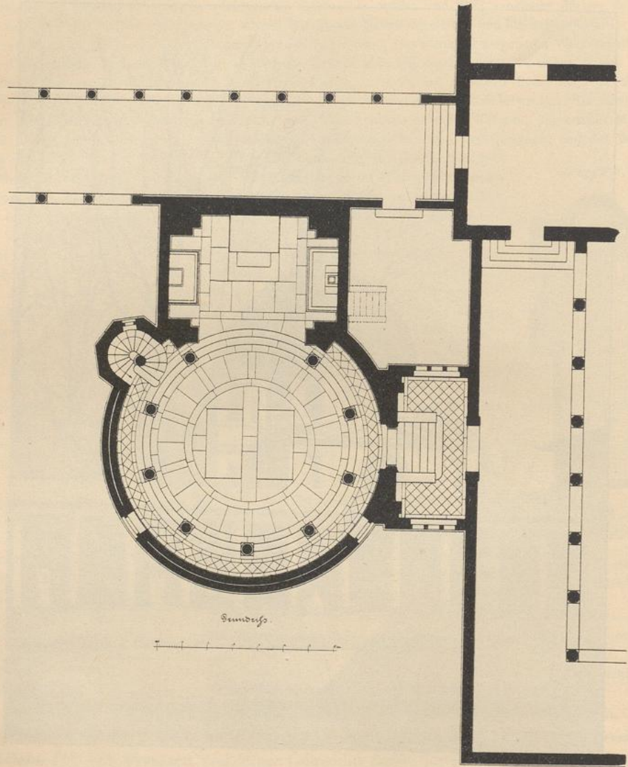
Kaiser Friedrich III. Mausoleum zu Potsdam. Grundriß (271). Arch.: J. C. Raschdorff.
