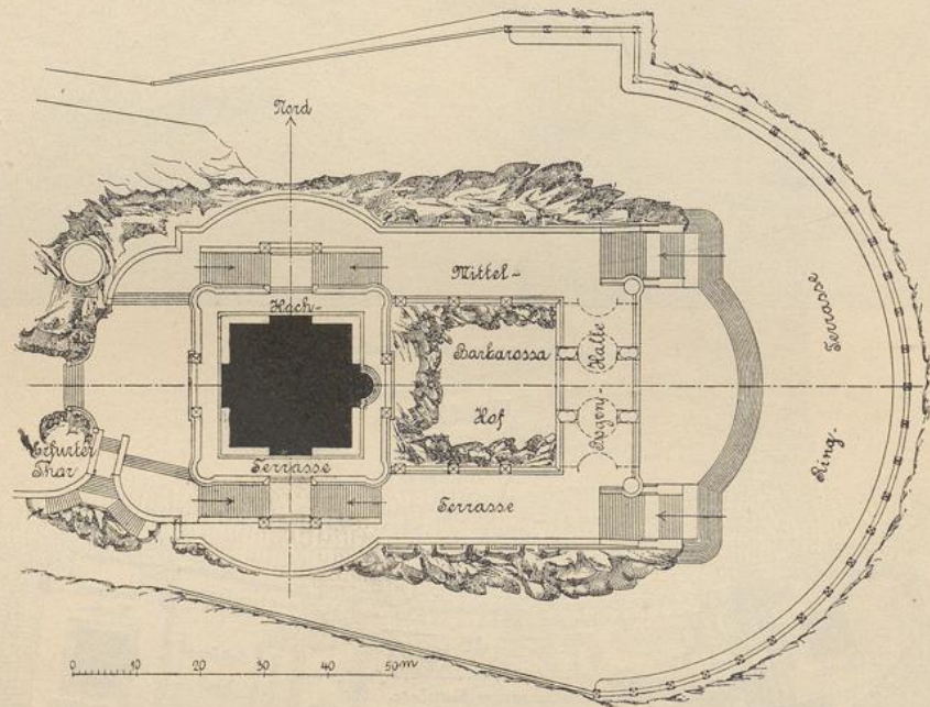
Grundriß des Kaiserdenkmals auf dem Kyffhäuser.
