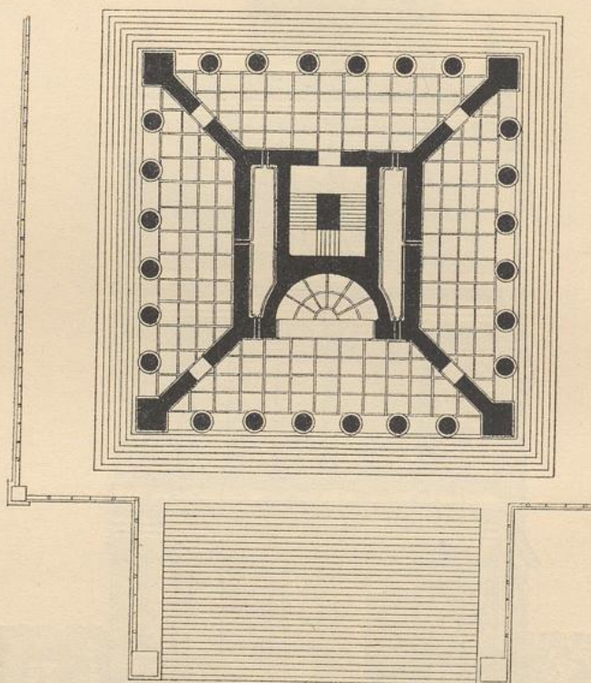
Grundriß zu Fig. 343.
