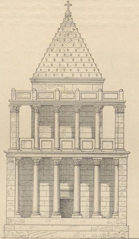
Anficht. — \frac{1}{200} w. Gr.
