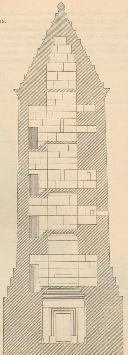
Lotrechter Schnitt.
