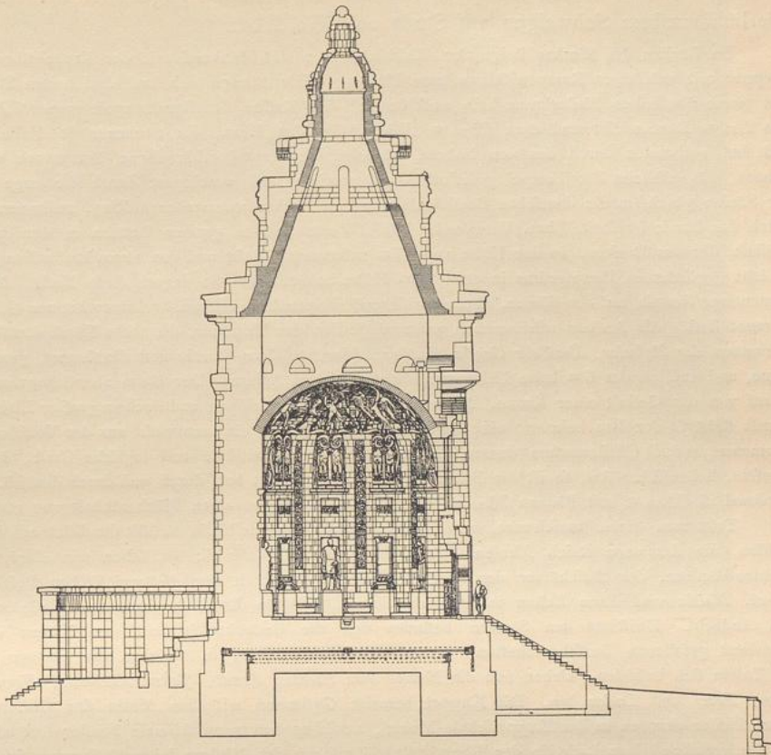
Lotrechter Schnitt.
