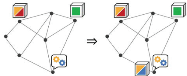
Bereitstellung heterogener Ressourcen (Boxen) mit gemeinsamer Instanziierung von Gütern (Farben) für Anfragen in einem Netz. Providing heterogeneous resources (boxes) with a joint instantiation of commodities (colors) for requests in a network.
