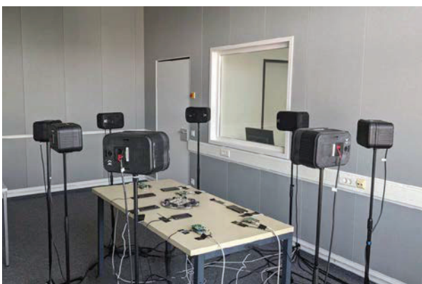
Experimentalaufbau für die Aufnahme simulierter Gesprächssituationen mittels verteilter Mikrofontgruppen. Experimental setup for the recording of simulated conversation situations using distributed microphone groups.
