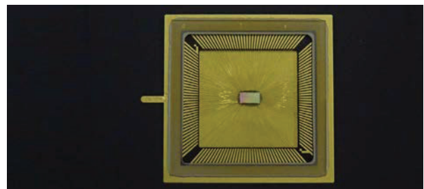
Gefertigter Scale4Edge-Ökosystem-Chip in 22FDX-Technologie mit Glasabdeckung
