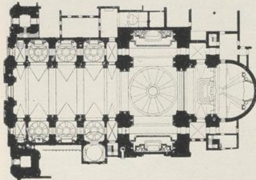
Abb. 78. St. Cajetan. Theatiner Hofkirche. Grundriß.
