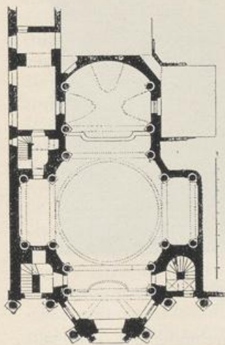
Abb. 109. Die Dreifaltigkeits- kirche. Von Gio. Anton. Viscardi. 1714. Nach den Kunstdenkmälern des Königreichs Bayern.
