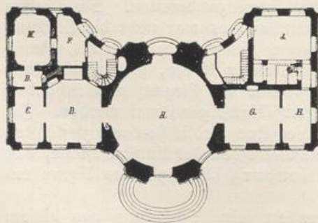
Abb. 96. Amalienburg. Grundriß. Nach Aufleger und Trautmann, Amalienburg.
