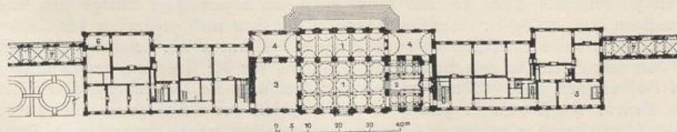
Abb. 85. Schleißheim. Grundriß des Erdgeschosses. Nach Streiter, Schleißheim und Nymphenburg.
