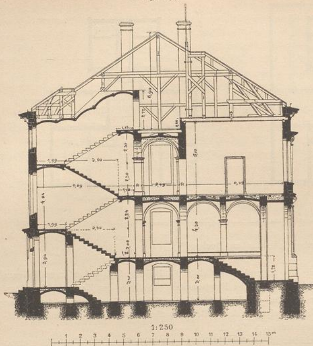
Querschnitt.
