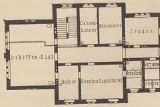
Obergeschoss.
