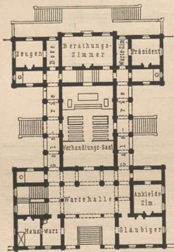
Erdgeschofs. — 1/500 n. Gr. Gerichtshaus zu Nyons 199) . Arch.: Bulot.
