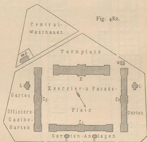
Cafernement des Kaiser-Franz-Garde-Grenadier-Regimentes zu Berlin 509) . — 1/5000 n. Gr.
