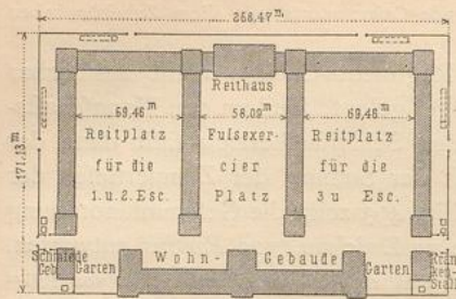
Caferne für das 2. Garde-Ulanen-Regiment zu Moabit 510) . — 1/5000 n. Gr. Arch.: Drewitz.
