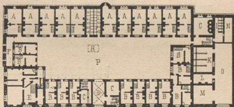
Miliz-Caferne zu Chester. — 1/1000 n. Gr.
