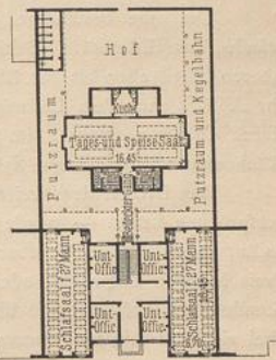
Guillaume's Entwurf für das Compagnie-Revier einer englischen Infanterie-Caferne.
