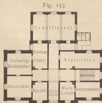
Erdgeschoss. — 1/500 n. Gr. Amtsgerichtshaus zu Neckar- bifchofsheim 187).
