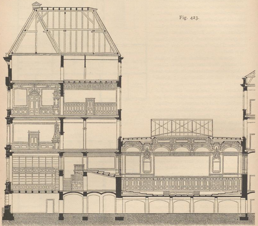
Landeshaus der Provinz Brandenburg zu Berlin. — Querschnitt 463 ).
