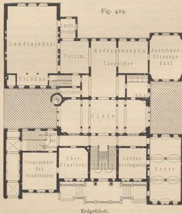
Landeshaus der Provinz Westpreußen zu Danzig 460) .
