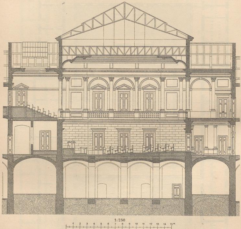
Landhaus zu Brünn. — Schnitt nach der Hauptaxe des Sitzungsfaales 455) .
