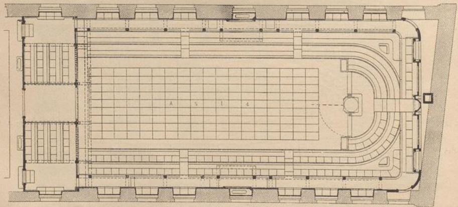
Grundriß.
