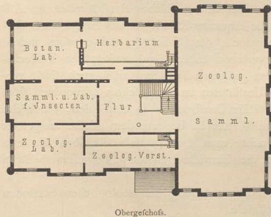
Obergeschofs.
