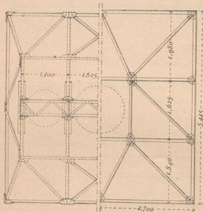
Glockenstuhl zu Neuenkirchen. \frac{1}{100} n. Gr.
