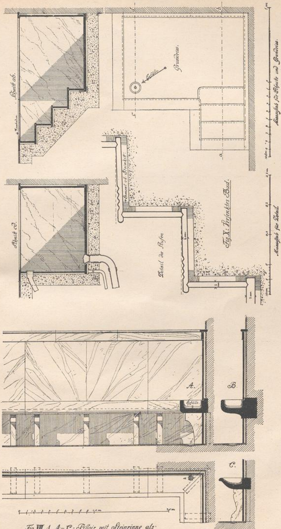
Fig. VIII. 1. A—C: Pissoir mit Steinrinne als Ersatz für die Urinale.
