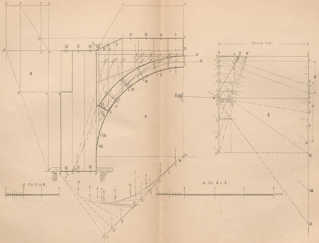
Stabilitäts-Untersuchung eines symmetrischen Tonnengewölbes und seines Widerlagers.
