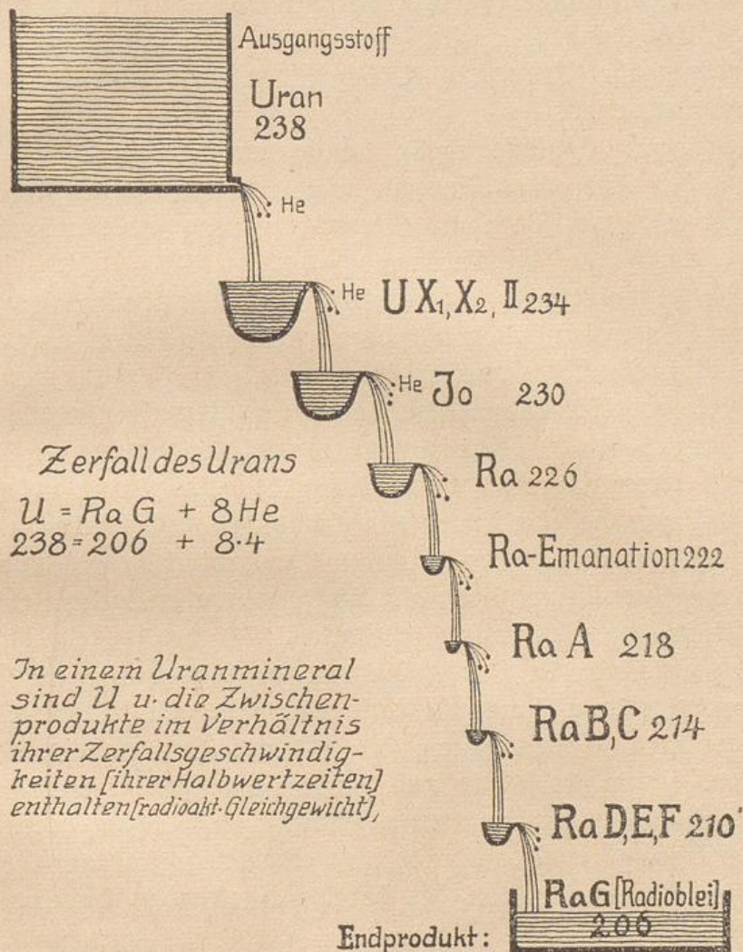
Abb. 20. Die Uranuhr.
