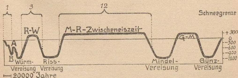
Abb. 5. Klimakurve der Eiszeit nach Penck. A Achenschwankung (Rückzug der Gletscher). B Bühlovorstoß.
