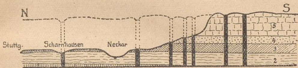
Abb. 2. Querschnitt durch die Schwäbische Alb und ihr Vorland mit vulkanischen Durchschlagsröhren. Zur Zeit der Eruption muß noch eine Gesteinsdecke, wie sie durch die gestrichelte Linie angedeutet ist, über dem Vorland gelegen haben. 1 Muschelkalk, 2 Keuper, 3 Schwarzer Jura, 4 Brauner Jura, 5 Weißer Jura.
