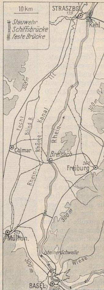
608. Der Oberrhein von Basel bis Straßburg.
