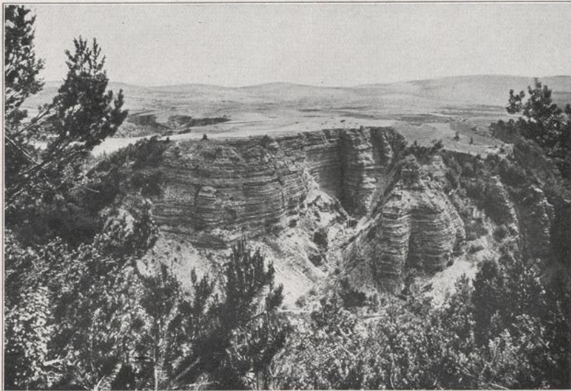
624. Die Causses: Le Bramabiau. Über 1000 m hoch liegen die Kalktafeln der Causses auf dem südlichen Zentralplateau. Im Hintergrund die rundlichen Hügel des kristallinen Gebirges, davor die nur zur Schafweide dienenden Kalkhochflächen. Im Vordergrund die großartigen Schluchten der in die Kalktafeln eingesenkten Täler.
