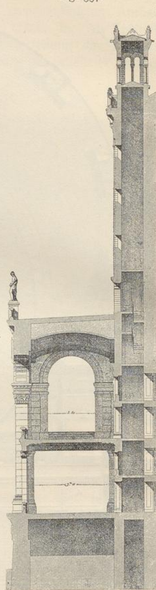
Trocadéro-Palast zu Paris 242 .
