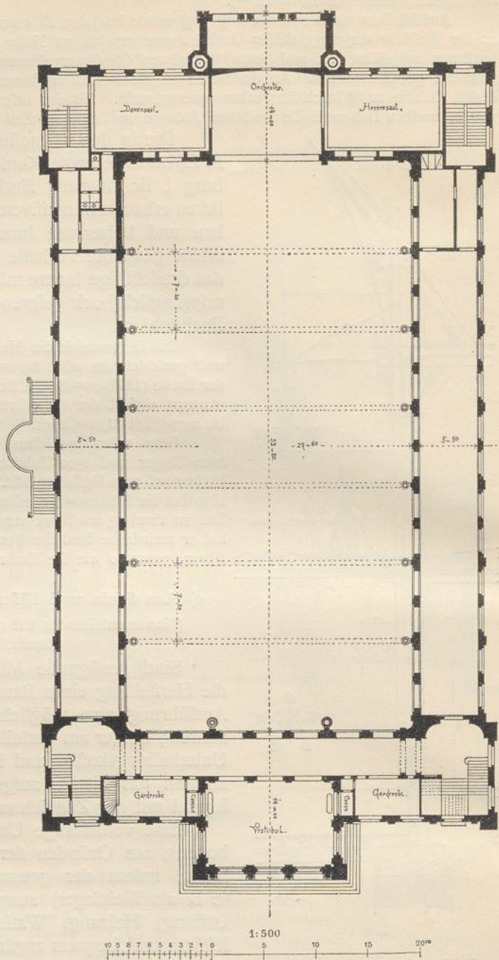
Stadthalle zu Mainz 233) .
