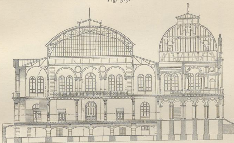
Schnitt durch die Gewerbehalle zu Stuttgart 236 ).
