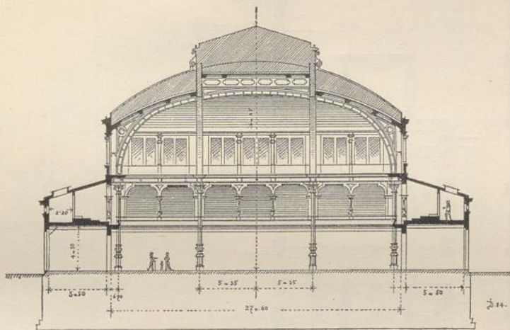
Querschnitt der Stadthalle zu Mainz 233 ).
