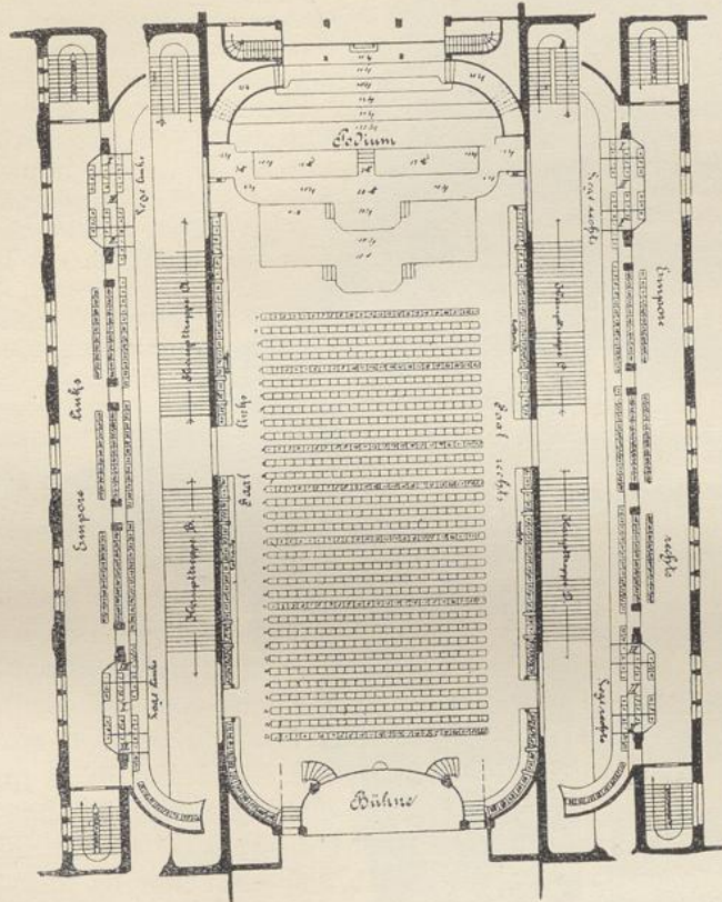
Festsäle zu Mannheim.
