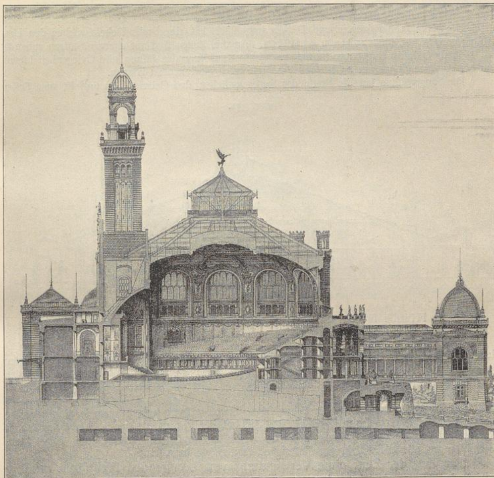
Längenschnitt des Festsaales im Trocadéro-Palast zu Paris 242) .
