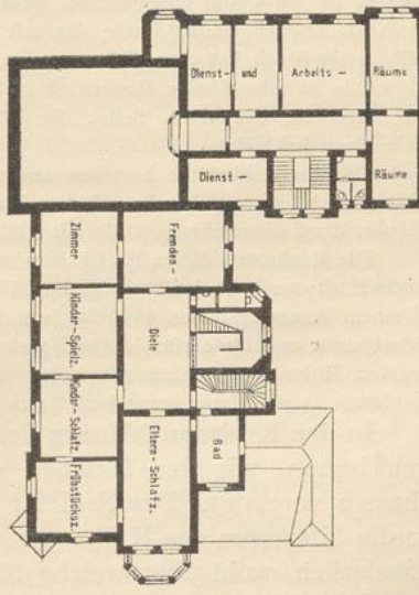
I. Obergeschoss.
