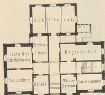
Erdgeschofs. — 1/500 w. Gr. Amtsgerichtshaus zu Neckar- bischofsheim 313) .
