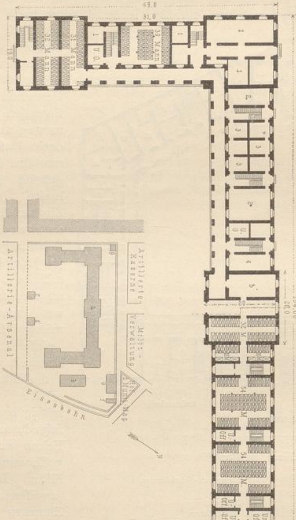
Fig. 104. Erdgeschoss. 1. Magazine. 2. Stallungen. 3. Wohnungen der Werkstättenmeister. 4. Rapportzimmer. 5. Tanzsahl. a. Hauptgebäude. b. Küchengebäude und Arresthaus. c. Kasernenwärter.
