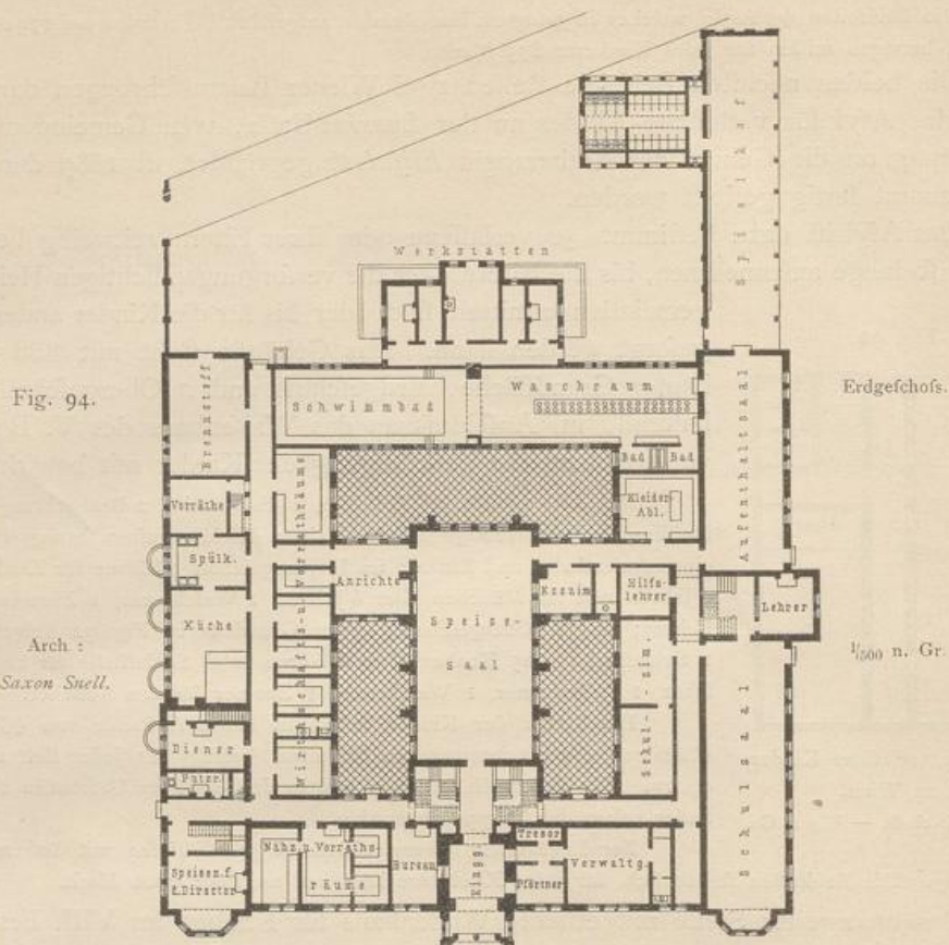
Waifenhaus für Soldatenkinder zu London 65) .
