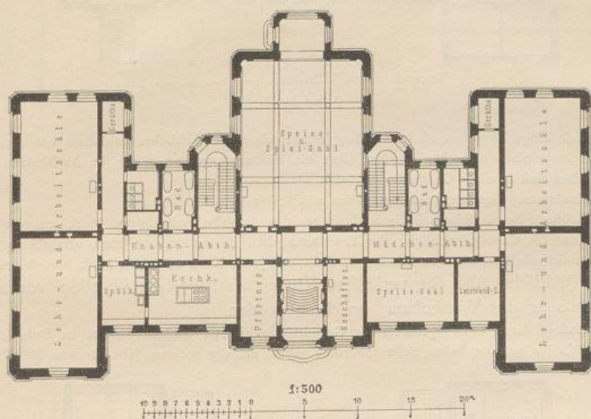
Städtisches Kinder-Afyl zu München. — Erdgeschoss.
