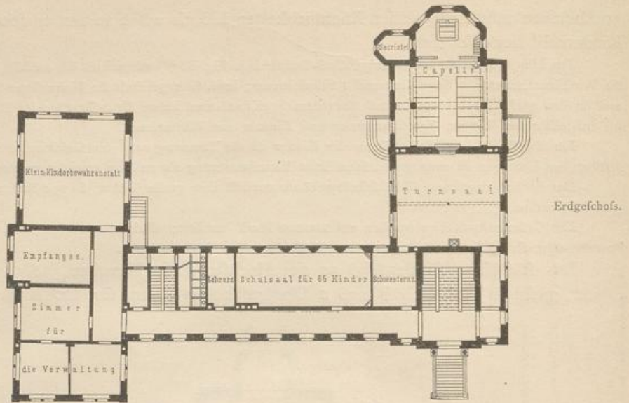
Vincentinum zu Würzburg. — 1/800 n. Gr.
