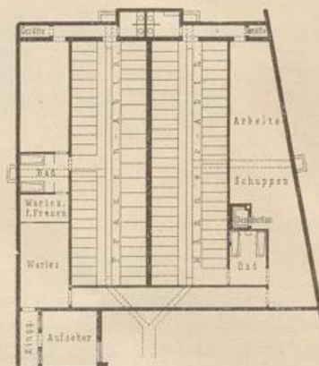
Afyl für Obdachlose zu London, Northumberland-Strafsse. Erdgeschofs 76) . — 1/500 n. Gr. Arch.: Saxon Snell .
