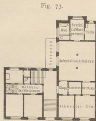
Krippe zu Hamburg-Hammerbrook. Maria-Apollonia -Krippe zu Düren. Erdgeschofs. Erdgeschofs. Arch.: Haftedt . Arch.: Schleicher .
