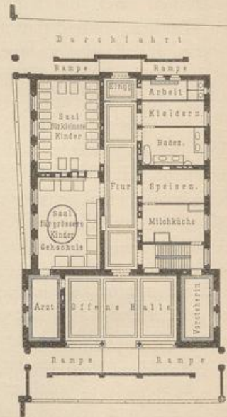
Krippe zu Hamburg-Hammerbrook. Maria-Apollonia -Krippe zu Düren. Erdgeschofs. Erdgeschofs. Arch.: Haftedt . Arch.: Schleicher .
