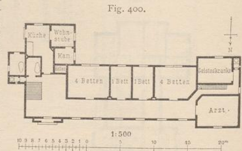
Kranken-Pflegehaus zu Wilster. Erdgeschofs 1755). 1869 u. 1879.
