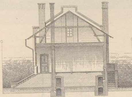
Querschnitt.
