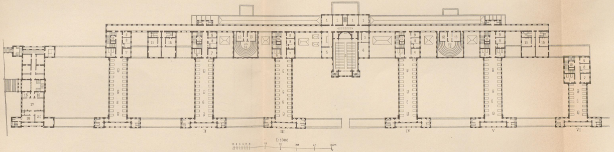
St. Thomas-Hospital zu London. I. Obergeschoß. 1866—71. Arch.: Currey.
