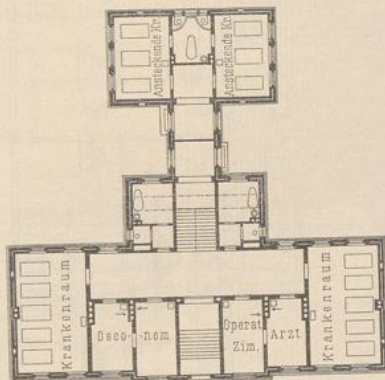
Städtisches Krankenhaus zu Neumünster 1753 ). 1888—89.
