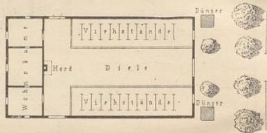
Altsächsisches Bauernhaus. 1/600 w. Gr.
