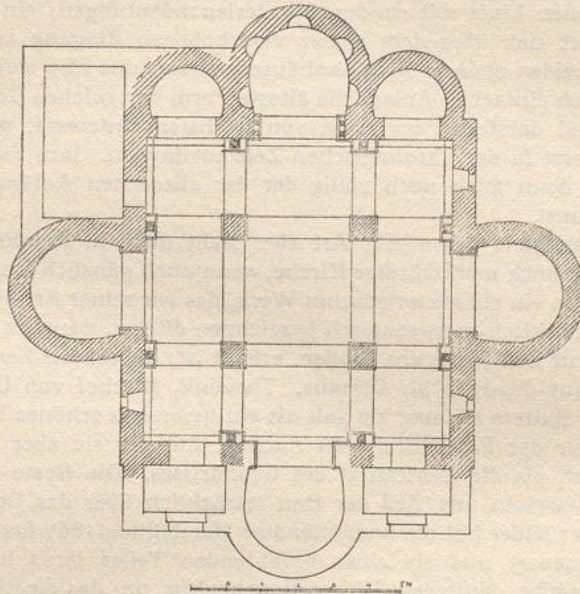
Abb. 160. Germigny-des-Prés. Grundriß.
