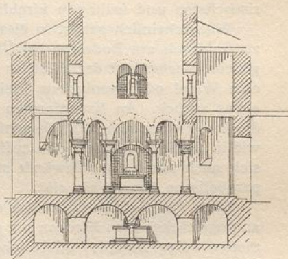
Abb. 176. Fulda. S. Michael. Schnitt.
