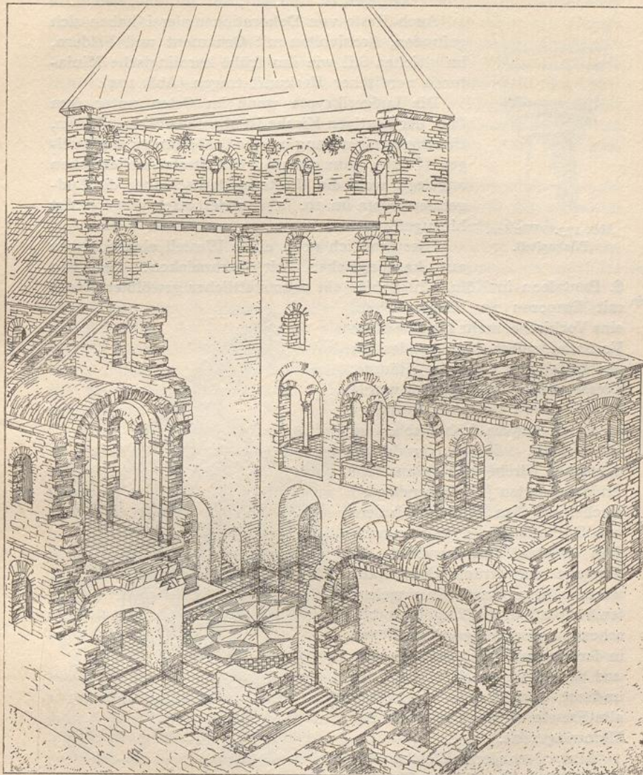
Abb. 172. Werden. Peterskirche. Perspektivischer Schnitt.
