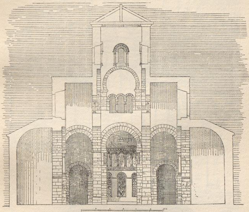
Abb. 161. Germigny-des-Prés. Schnitt.
