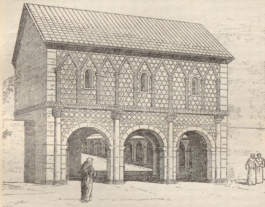
Abb. 149. Torhalle zu Lorsch. Nach Adamy.
